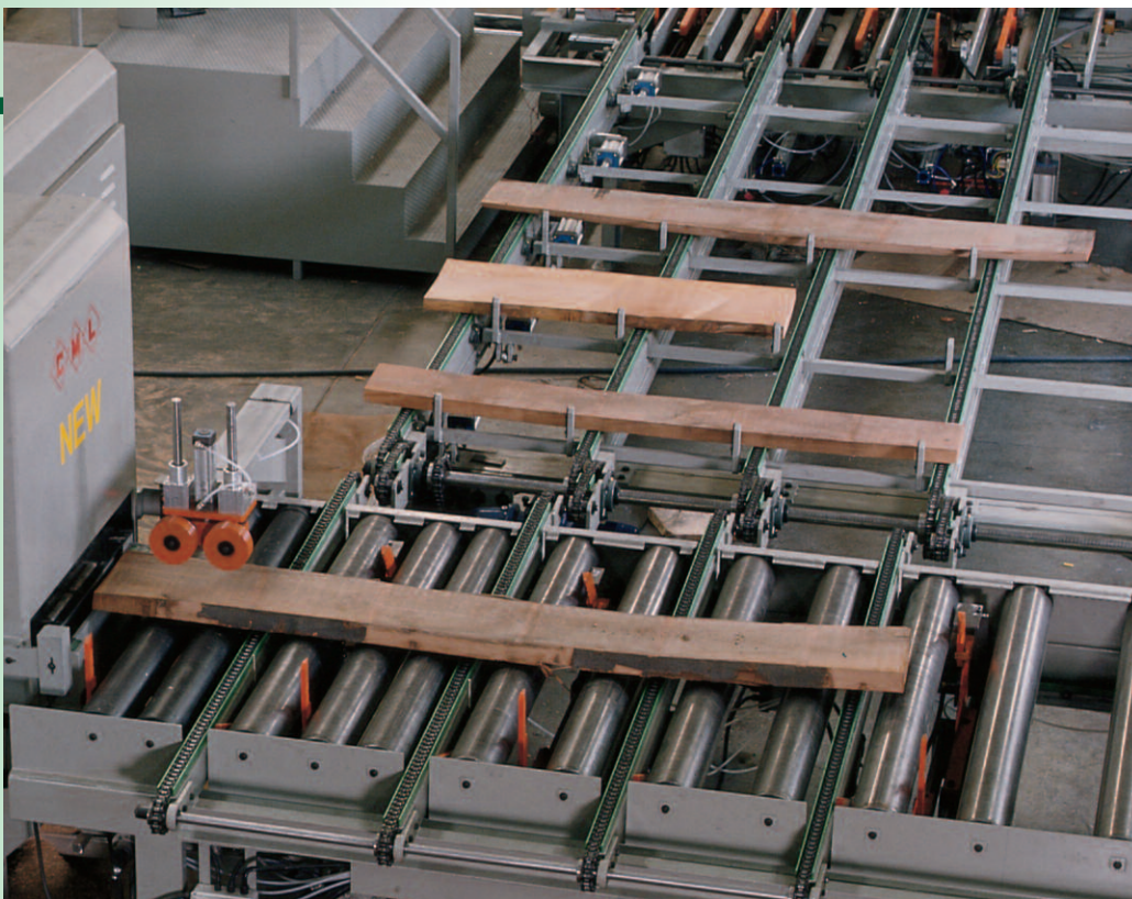
Trasportatore a catena con stoccaggio tavole in lavorazione.
