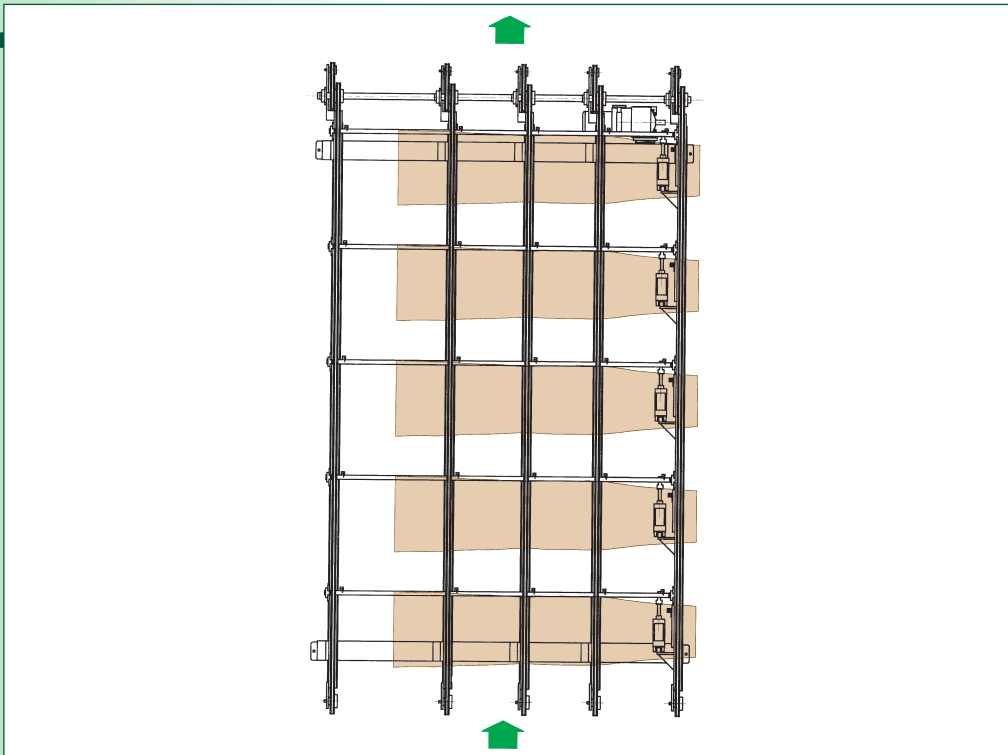
Trasportatore a catena con stoccaggio tavole in lavorazione.
